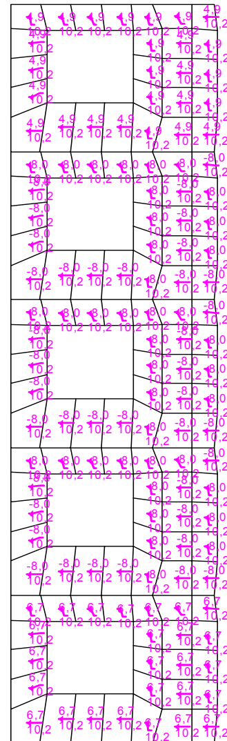
Рисунок 2. Пример задания температурной нагрузки: 2.а – задание численных параметров, 2.б – отображение на расчетной схеме
