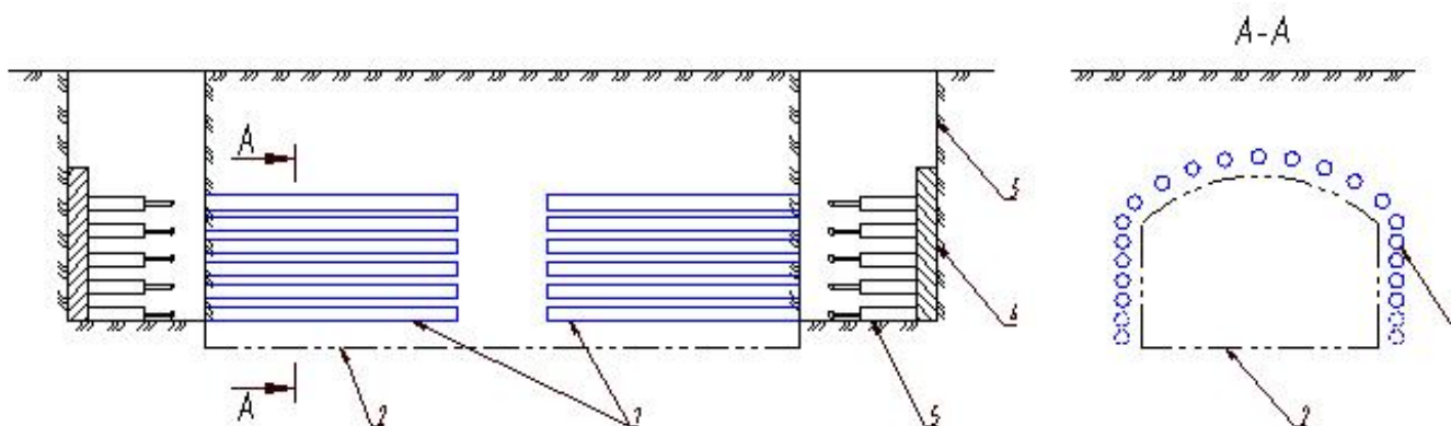
Рисунок 2. Схема экрана из труб: 1 – трубы; 2 – подземная выработка; 3 – котлован; 4 – упорная площадка; 5 – домкрат
