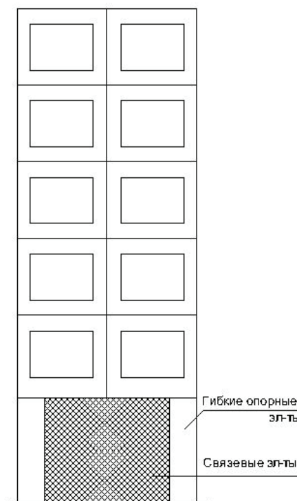
Рисунок 7. Пример конструктивного решения зданий с выключающимися связями
