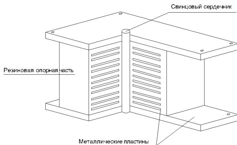
Рисунок 4. Антисейсмическая опора
