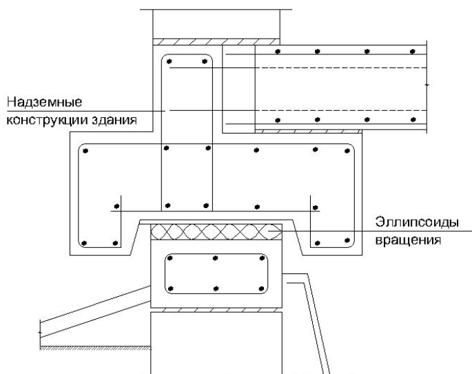
Рисунок 5. Сейсмоизоляционное устройство гравитационного типа
