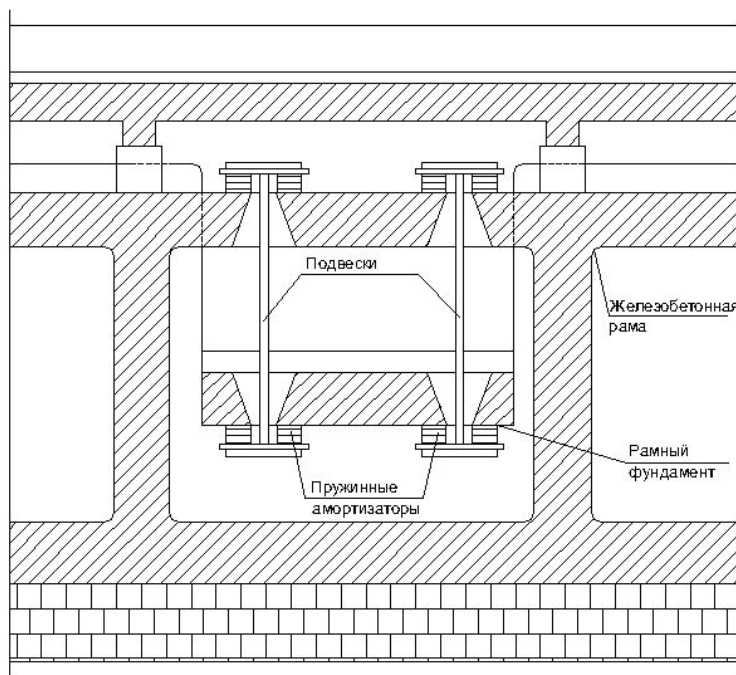
Рисунок 3. Схема фундамента подвесного типа
