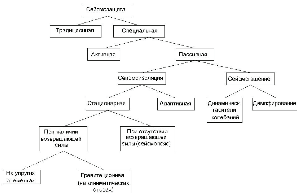
Рисунок 1. Классификация систем сейсмозащиты по принципу их работы
