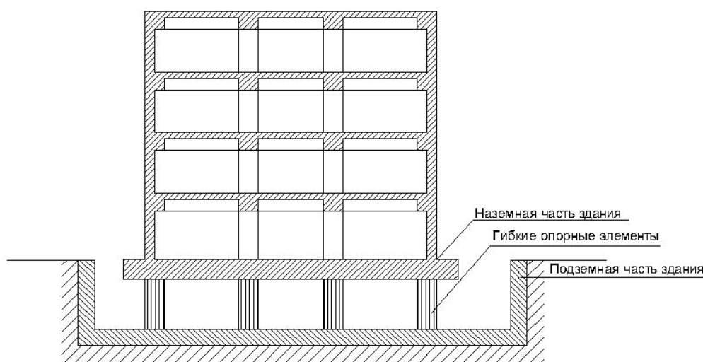
Рисунок 2. Здание с гибким нижним этажом
