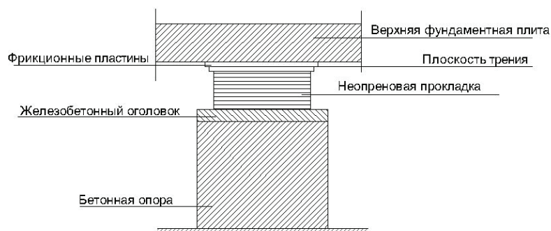
Рисунок 6. Сейсмоизолирующий фундамент фирмы Spie Batignolle
