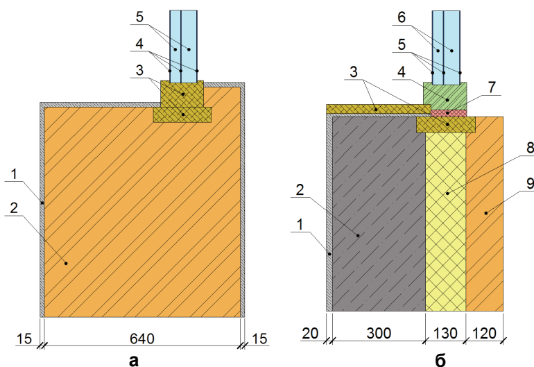
Рисунок 1. Схема расчетных узлов а – 1 вариант исполнения (1 – штукатурка; 2 – кладка из керамического кирпича; 3 – дерево (сосна поперек волокон); 4 – стекло оконное; 5 – воздушная прослойка); б – 2 вариант исполнения (1 – штукатурка; 2 – газобетон; 3 – дерево (сосна поперек волокон); 4 – утепленная оконная коробка; 5 – стекло оконное; 6 – воздушная прослойка; 7 – монтажная пена; 8 – изоляция Rockwool FASAD BATTS; 9 – облицовочный кирпич)
