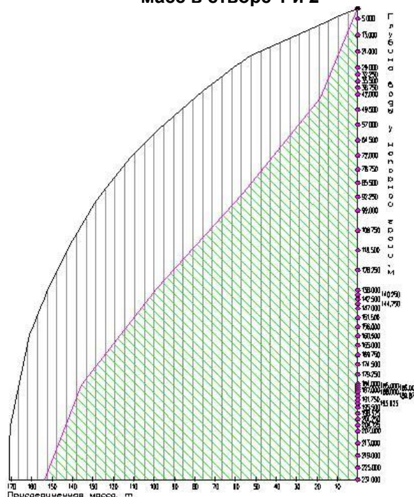
Рисунок 6. Эюра распределения точечных масс в створе 5 и 6
