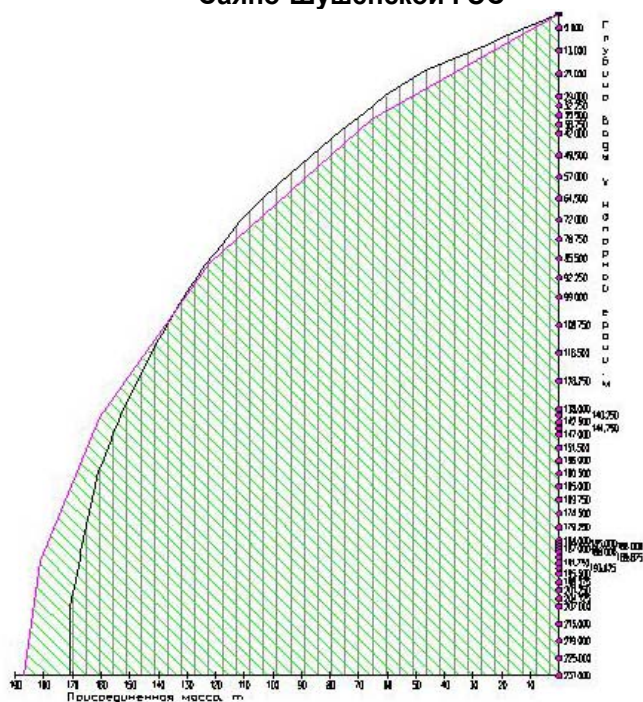
Рисунок 5. Эюра распределения точечных масс в створе 3 и 4
