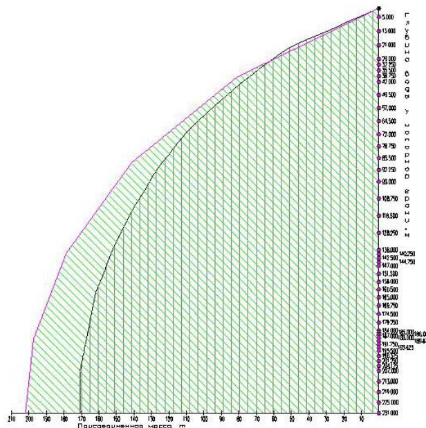
Рисунок 4. Эюра распределения точечных масс в створе 1 и 2
