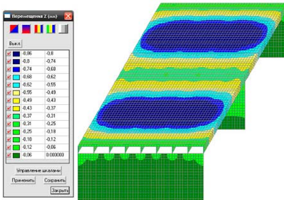
Рисунок 6. Деформации перекрытия
