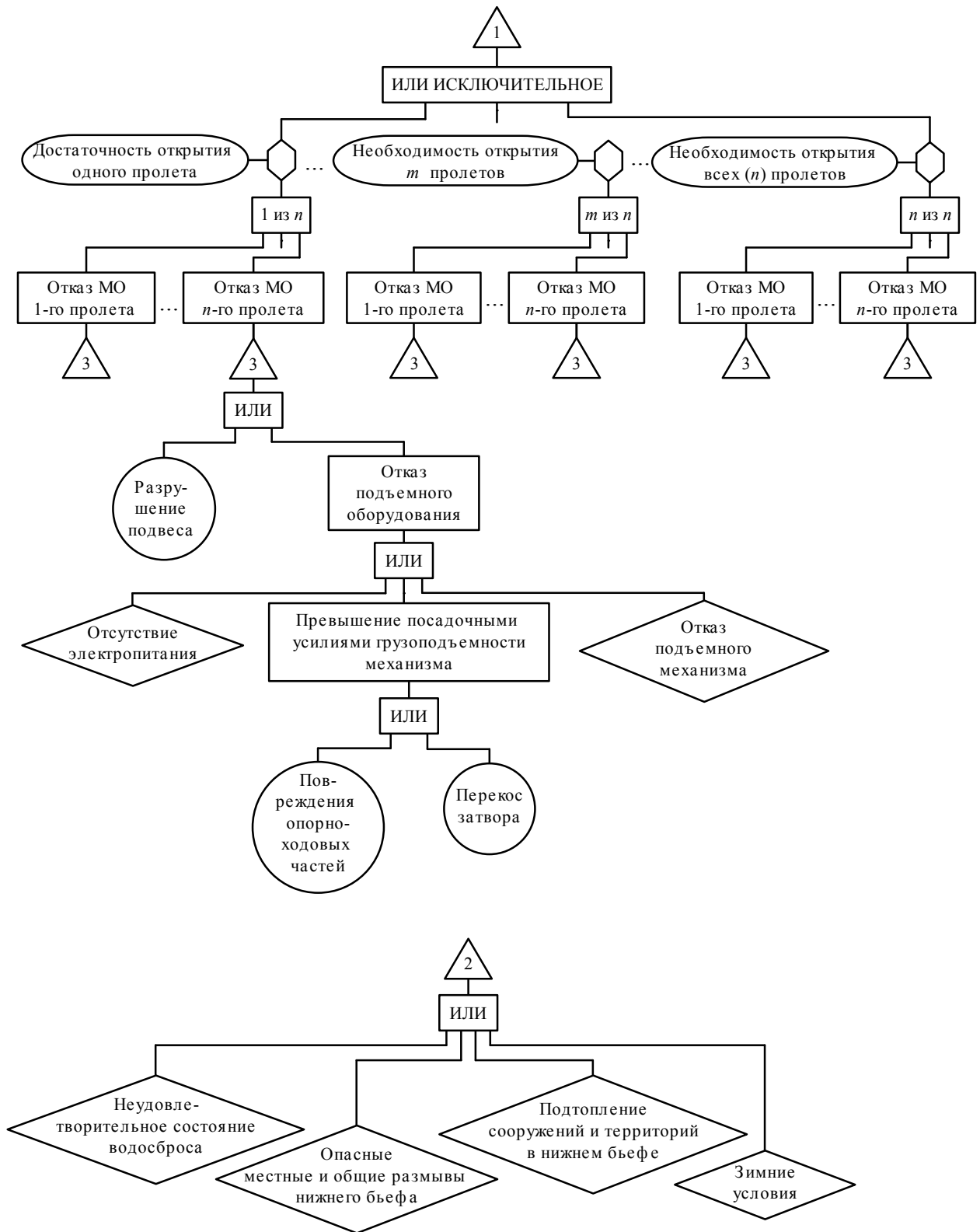
Рисунок 1. Дерево отказов, приводящих к переливу воды через гребень плотины вследствие недостаточной пропускной способности водопроводящих трактов (окончание)
