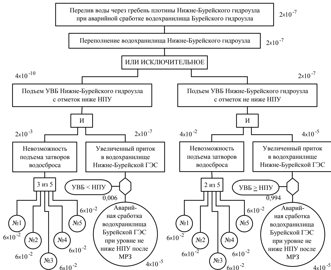
Рисунок 2. Расчет дерева отказов перелива воды через гребень плотины Нижне-Бурейской ГЭС при аварийной сработке водохранилища Бурейского гидроузла
