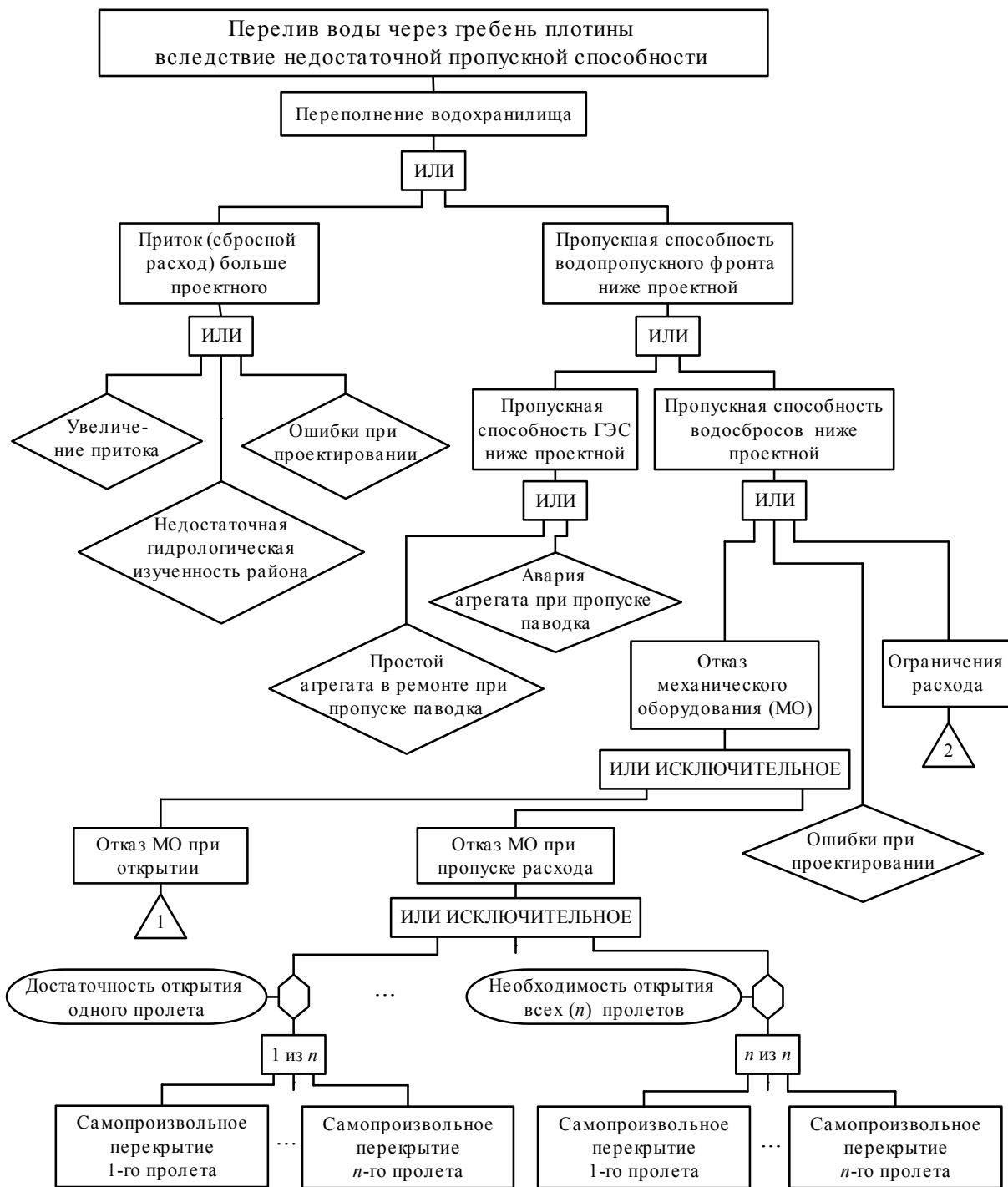
Рисунок 1. Дерево отказов, приводящих к переливу воды через гребень плотины вследствие недостаточной пропускной способности водопроводящих трактов (начало)
